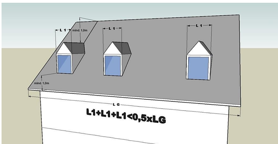
Bild 1: Schema Dachaufbauten
